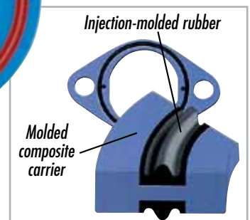
PermaDryPlus® Gasket
