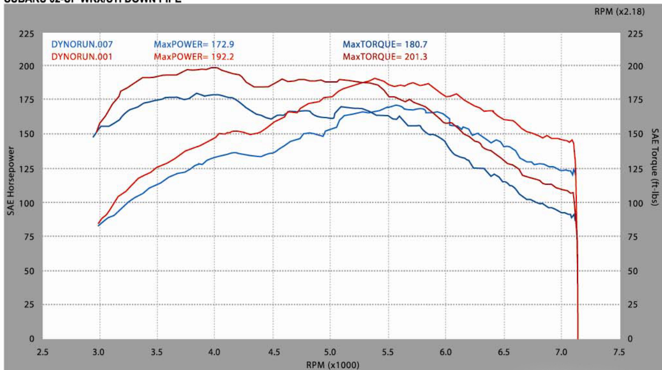
SUBARU 02-UP WRX/STI DOWN PIPE
