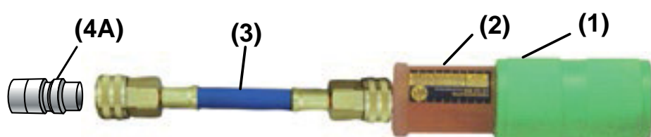
Mini Disposable Cartridge Type Injector (1 oz) 53809
