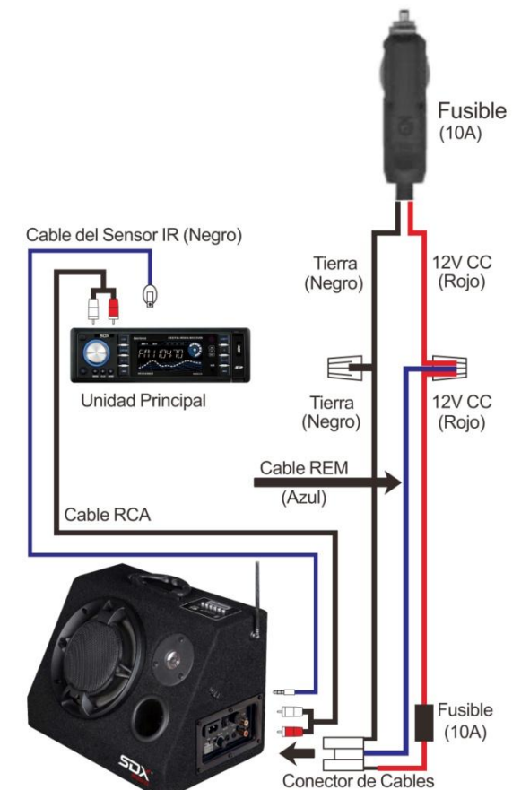
Diagrama rápido de cableado
