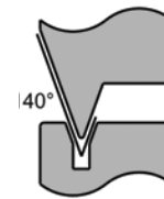
Hem Step #2 201-060-SK
